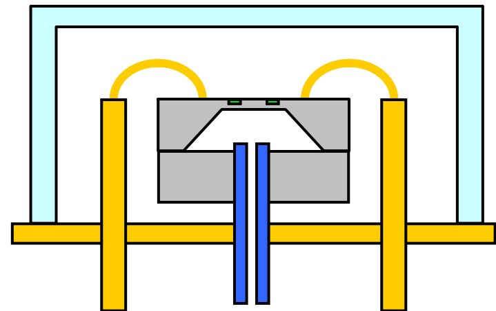
Sensor de pressão encapsulado
