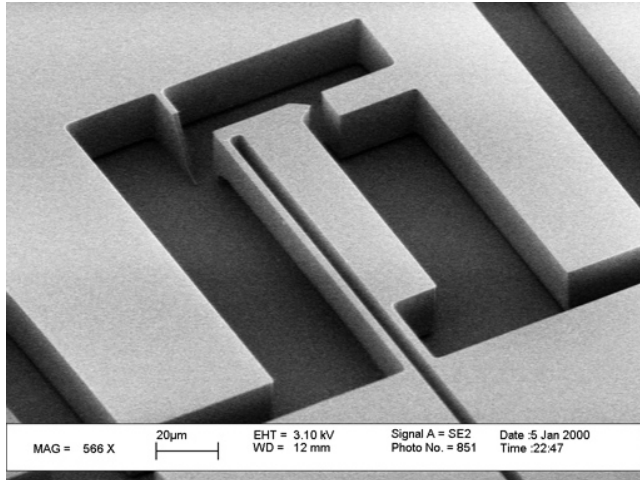
Actuador térmico
